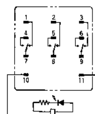
AC-Modell
