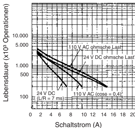
Lebensdauer
