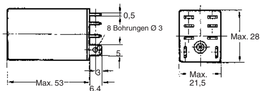
Modell: LY2N-CR
