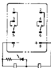
DC-Modell LY2(Z)N
