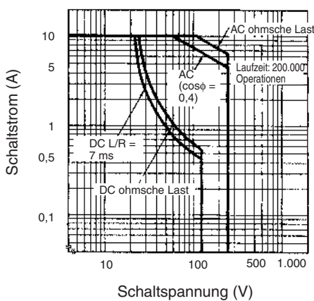
Maximale Schaltleistung
