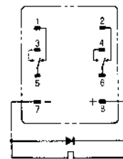
LY2(Z)-D
