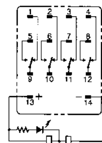
MY4(Z)N1/MY4(Z)IN1 (Nur DC-Modelle)
