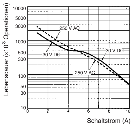
MY2 (ohmsche Lasten)
