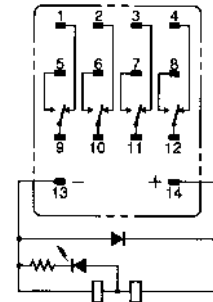
MY4(Z)N1-D2/MY4(Z)IN1-D2 (Nur DC-Modelle)
