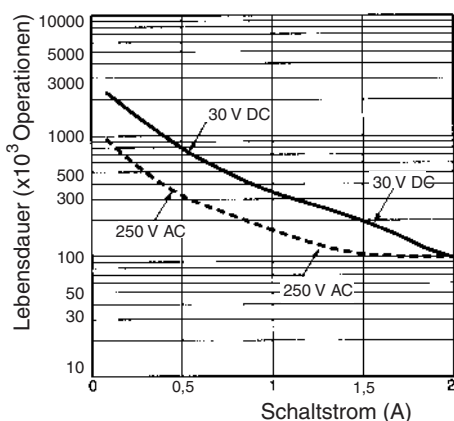
MY4 (induktive Lasten)
