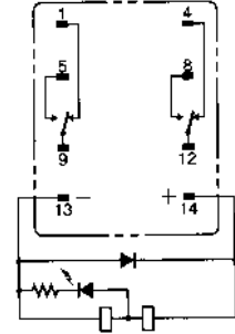
MY2N1-D2/MY2IN1-D2 (Nur DC-Modelle)
