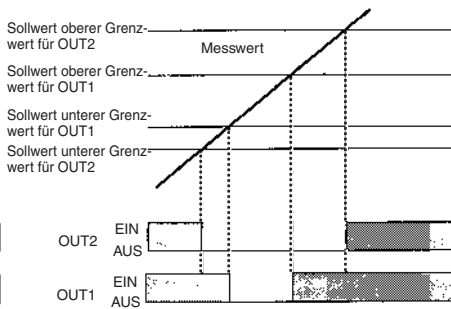
Schwellenwertausgang
