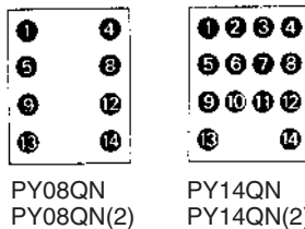
Klemmenbelegung (Ansicht von unten)
