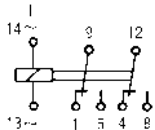
DIN-Schaltbild
