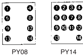
Klemmenbelegung (Ansicht von unten)
