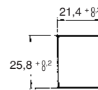
Schalttafelausschnitt
