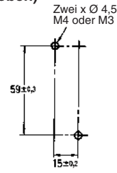
(Ansicht von oben)
