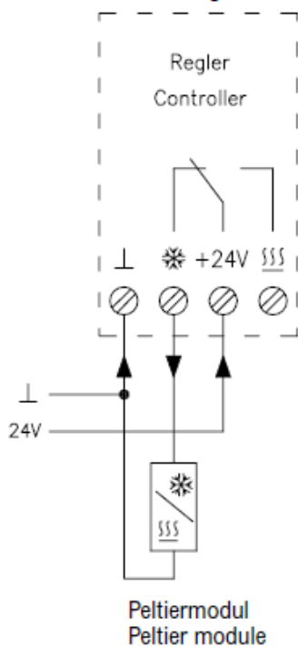
Anschluss im Kühlbetrieb Connection for cooling mode operation
