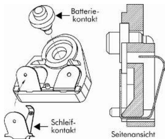
Bild 3: Skizze Federbügelkontakt in gemischter Technologie
